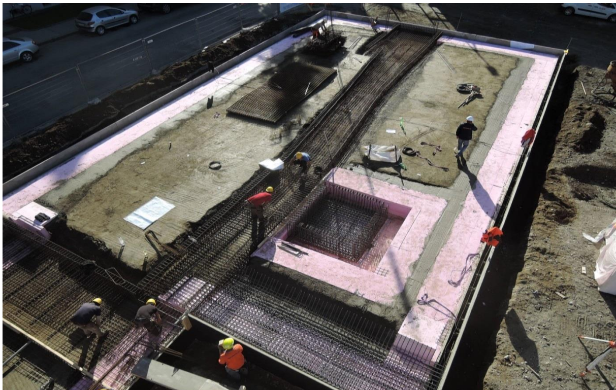
Studierenden-Wohnheim mineroom Detailplan Sockel und Fotos der Ausführung Dämmung unter der Bodenplatte. (Abb. und Fotos aap.architekten)
