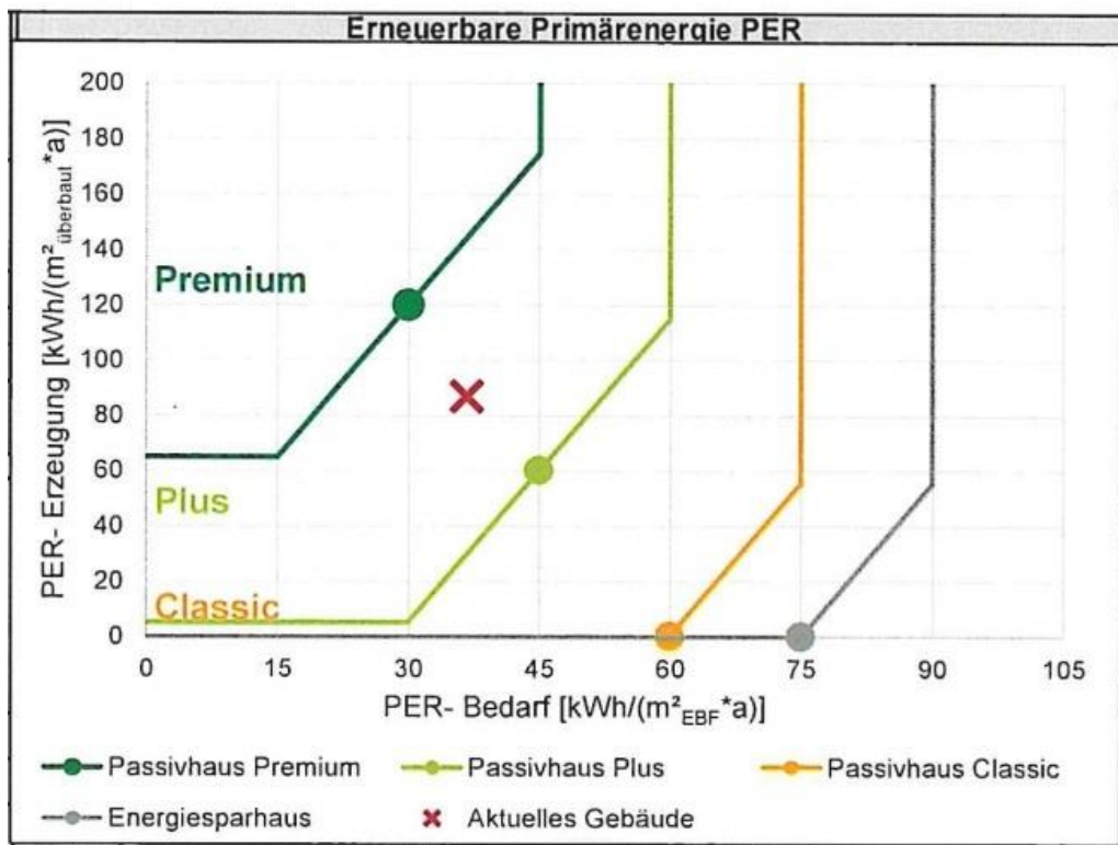
(Abb.: Schöberl & Pöll / Auszug aus PHPP_mineroom)
