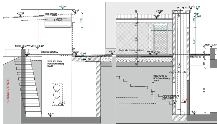
Studierenden-Wohnheim mineroom, Lüftungsbauwerk Frischluftansaugung. (Foto und Abb.: aap.architekten)
