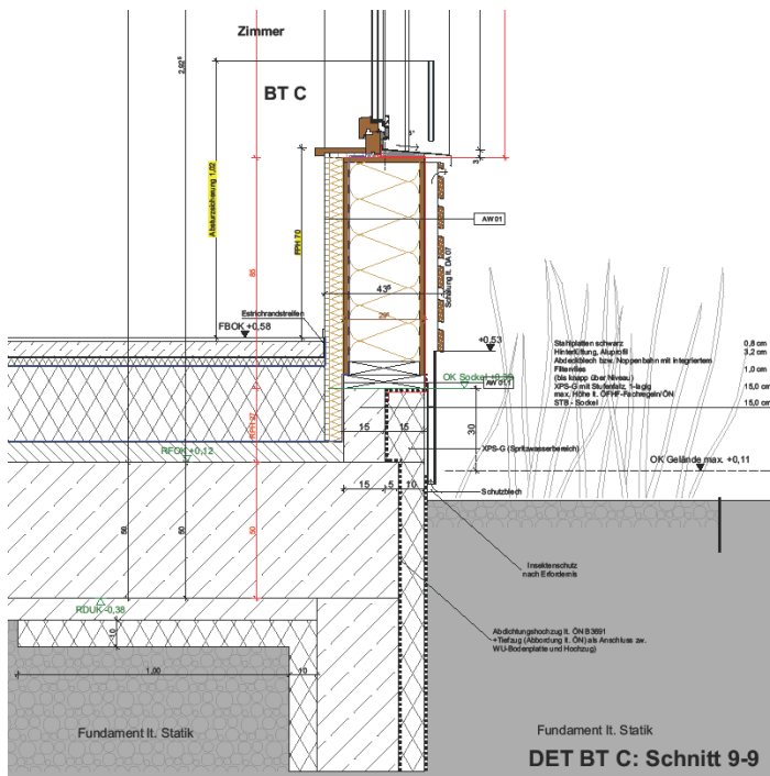
Studierenden-Wohnheim mineroom Detailplan Sockel und Fotos der Ausführung Dämmung unter der Bodenplatte. (Abb. und Fotos aap.architekten)
