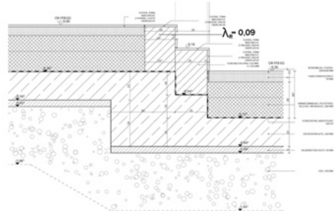
SCHICHTENAUFBAU - BODENPLATTE
